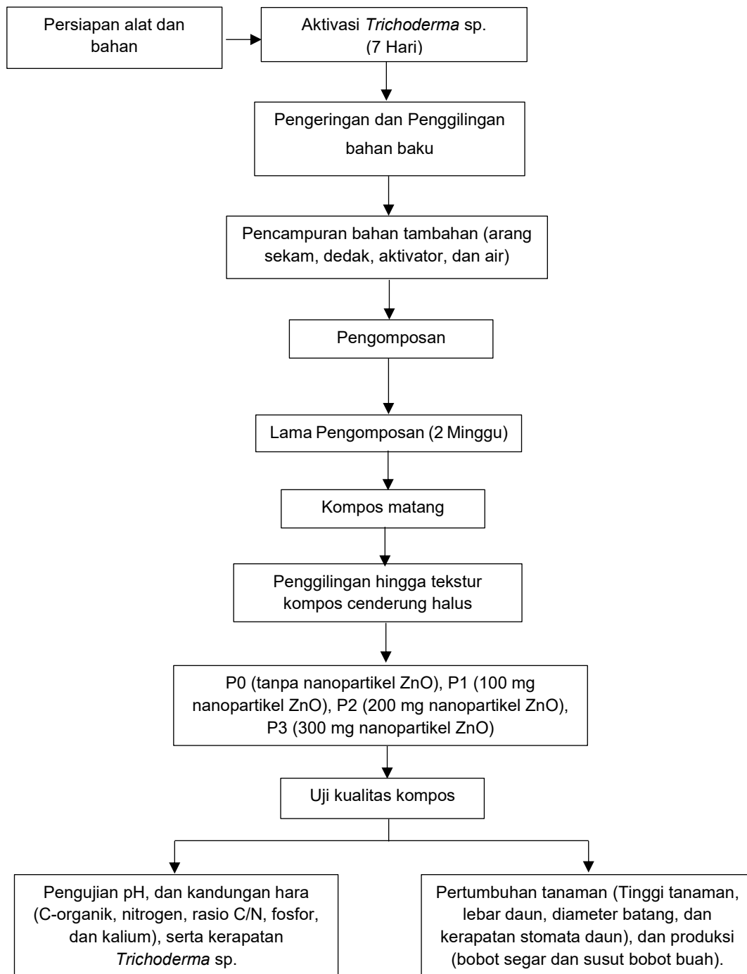
Gambar 3. Kerangka Operasional
